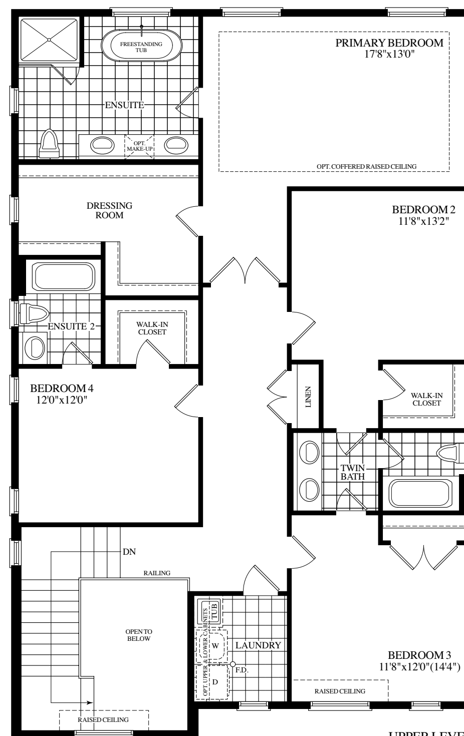
UPPER LEVEL ELEV.A
